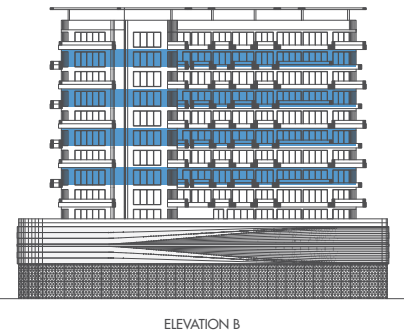
ELEVATION B
